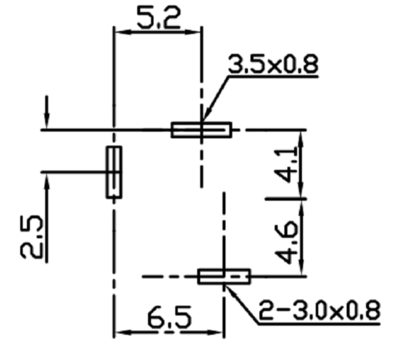
印制线路板开孔尺寸
